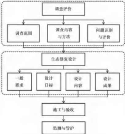
图 1 工作流程
